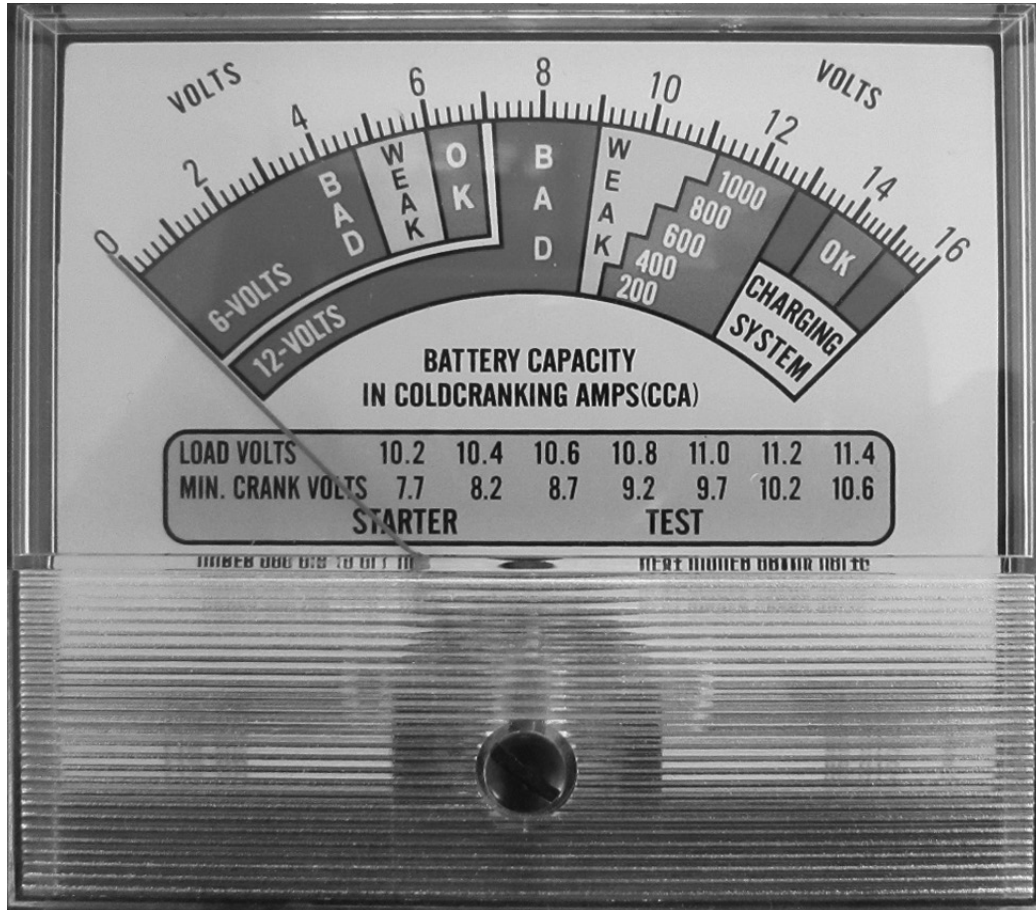
Meter Display
